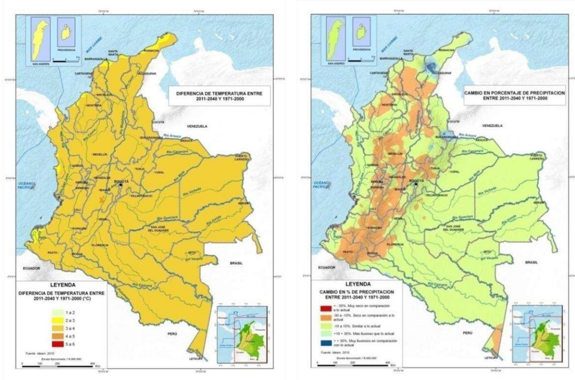
Figura (Der.) Mapa con el cambio en el porcentaje de precipitación del multimodelo del periodo 2011 a 2040 vs 1971 a 2000
