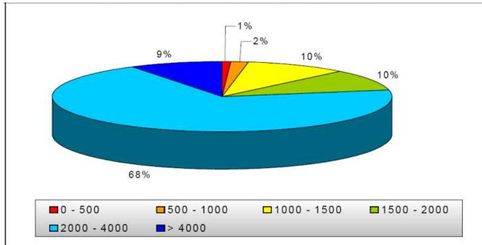
Figura 6.6 Precipitación anual en Colombia.
