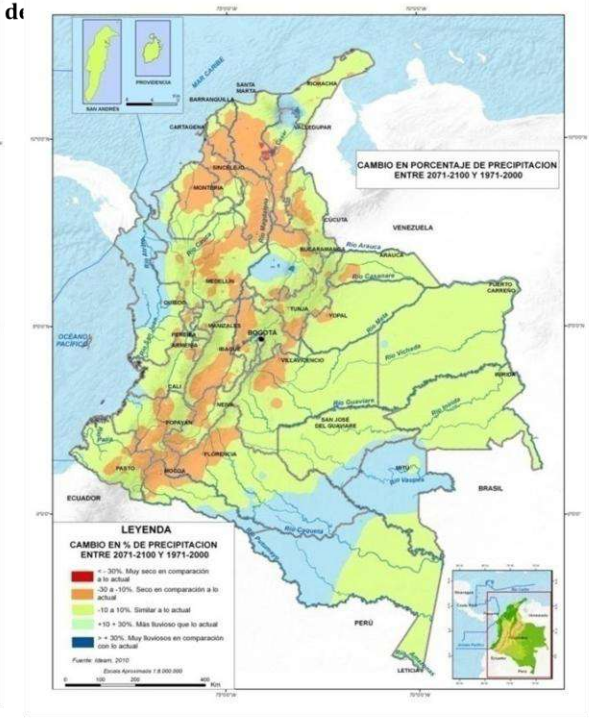
Figura (Der.) Mapa con el cambio en el porcentaje de precipitación del multi Diferencia Clasificación climatica Lang Actual vs Escenario 2011-2040 Coorporacion Autonoma Actual vs Escenario 1 Porcentaje Area CAM Similar 46 864117 Mas seco 54 1003230 Mucho mas seco 0 3939 1871286 CAR Similar 59 988317 Mas Humedo 0 31 Mucho mas humedo 0 20 Mas seco 41 675805 Mucho mas seco 0 1735 1665908 CORTOLIM A Similar 45 1088101 Mucho mas humedo 0 6 Mas seco 55
