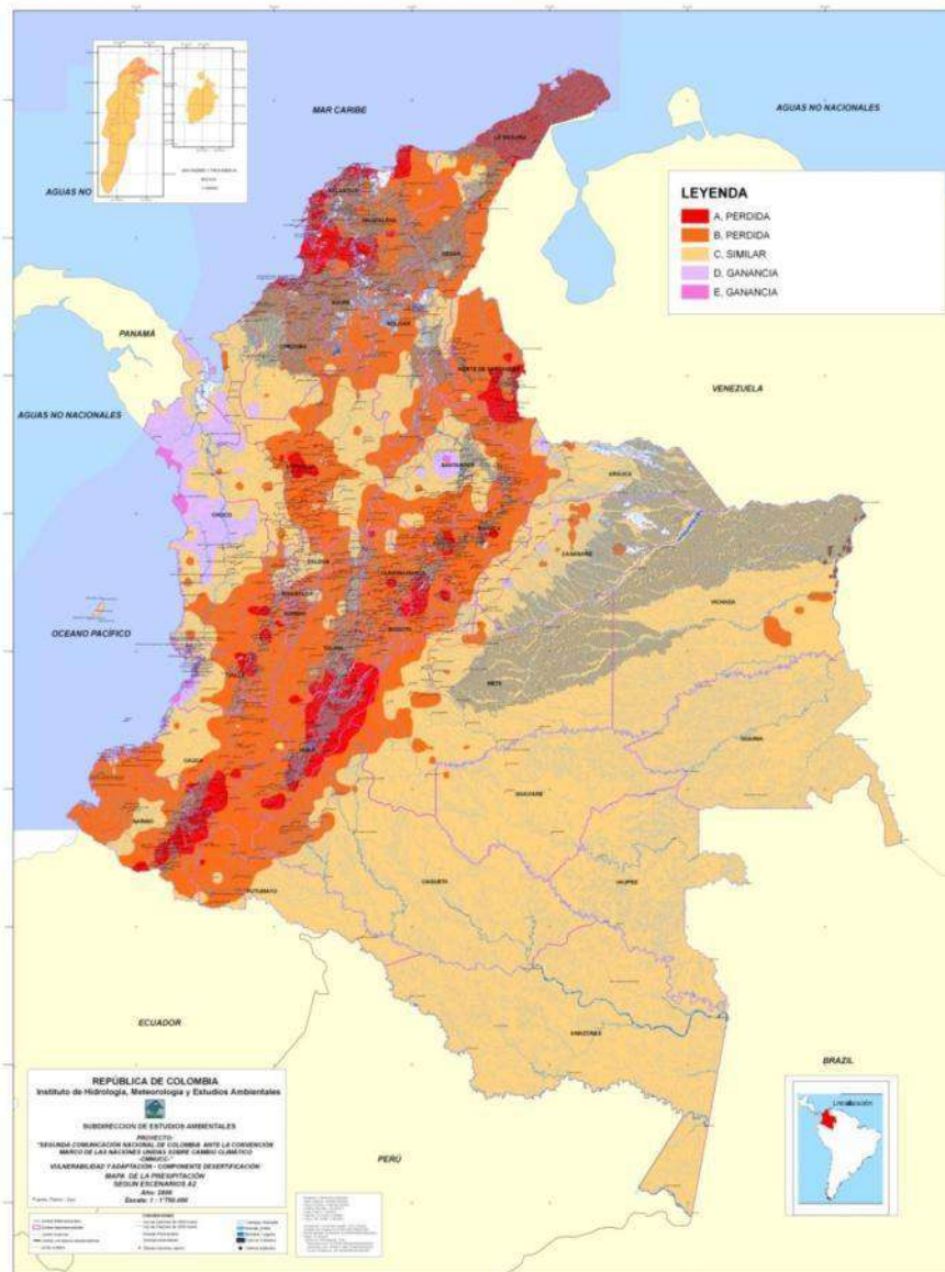
Mapa Cambios de la Precipitación en Colombia hacia el 2070-2100 (% del acumulado anual 1961-1990)
