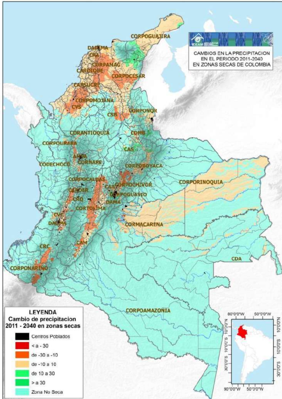
Figura 6.8 Escenario de precipitación 2011 – 2040 en zonas secas
