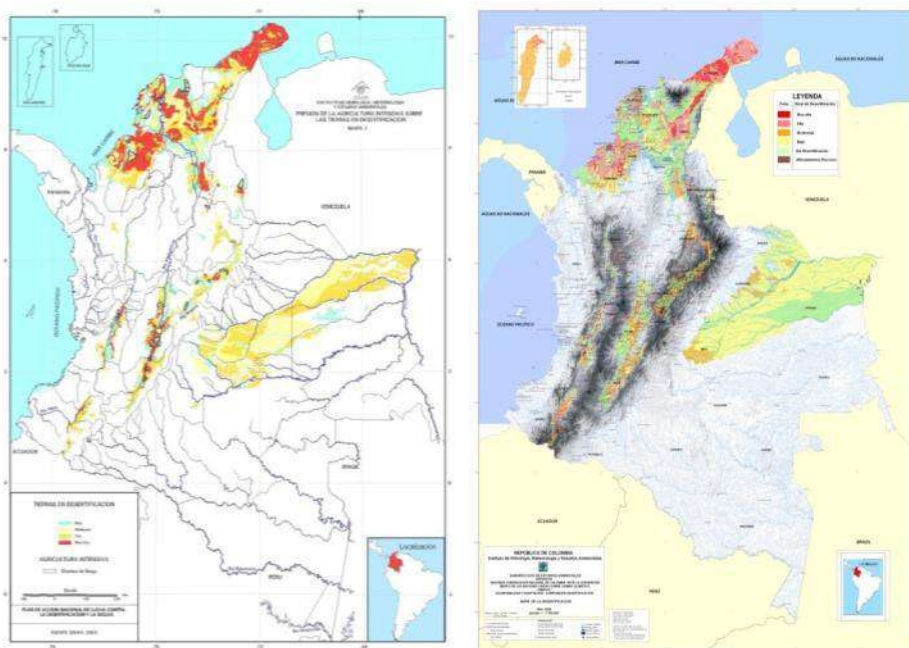
Figura 5.14 Tierras secas y en proceso de desertificación Izquierda. Elaborado en el año 2005. A la derecha. Elaborado en 2009 Fuente IDEAM
