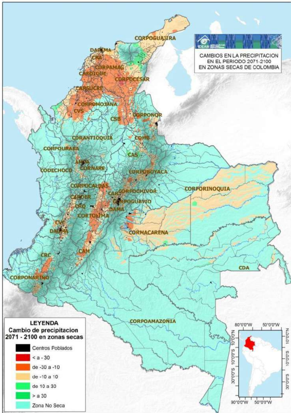
Figura 6.9 Escenario de precipitación 2071 -2100 en zonas secas
