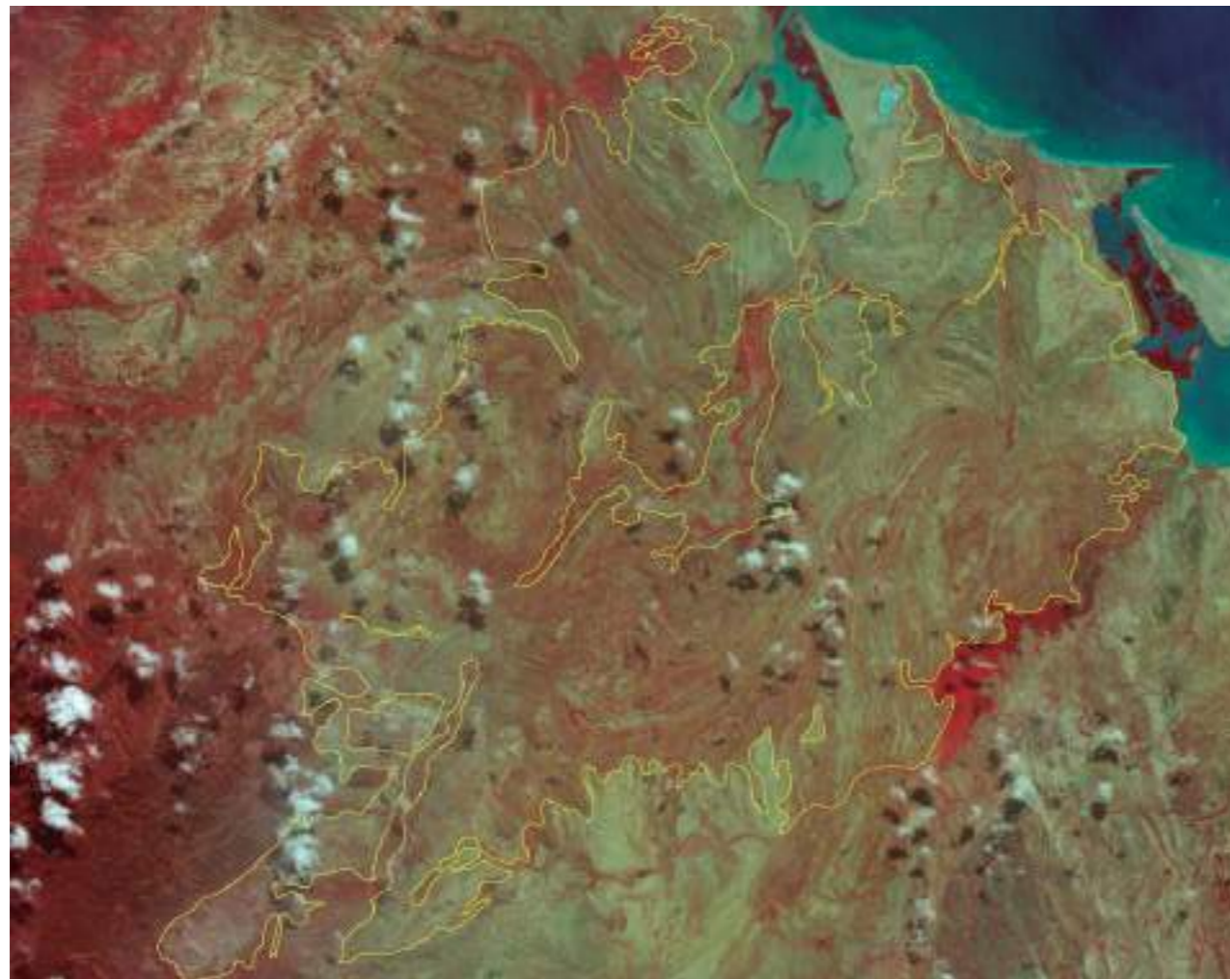
Figura 2.12. ~ Degradación de los suelos por erosión tipo eólica/clase pavimento del desierto/grado muy severa. Uribia (La Guajira). Apoyo de imagen satelital spot_648_326_050324_m_e. Combinación R,G,B: 1,2,3.
