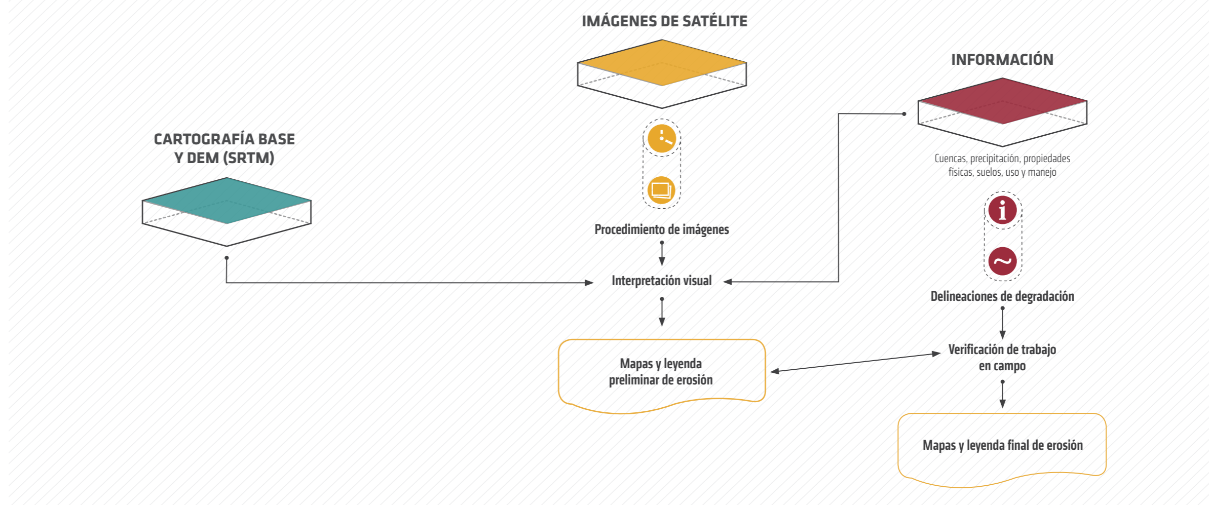
Figura 2.6. ~ Esquema metodológico para la zonificación de áreas degradadas por erosión por medio de interpretación de sensores remotos.
