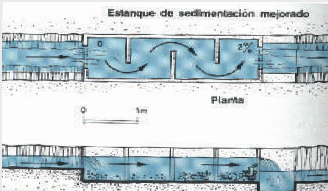
Figura 5 Estanque de sedimentación
